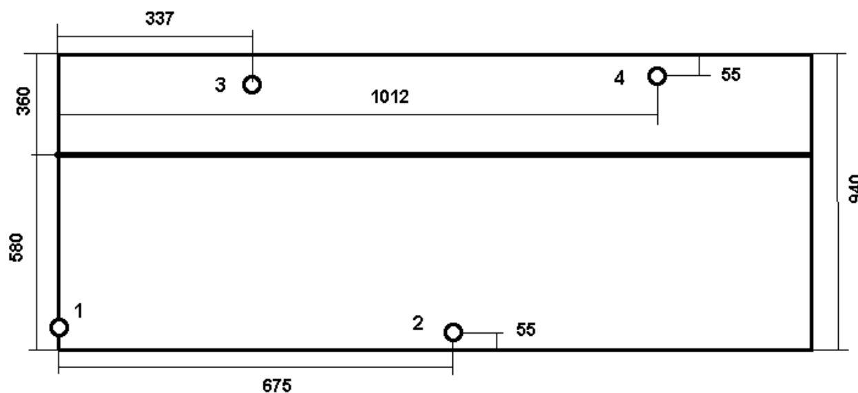
Рис. 7.8. Схема контроля
