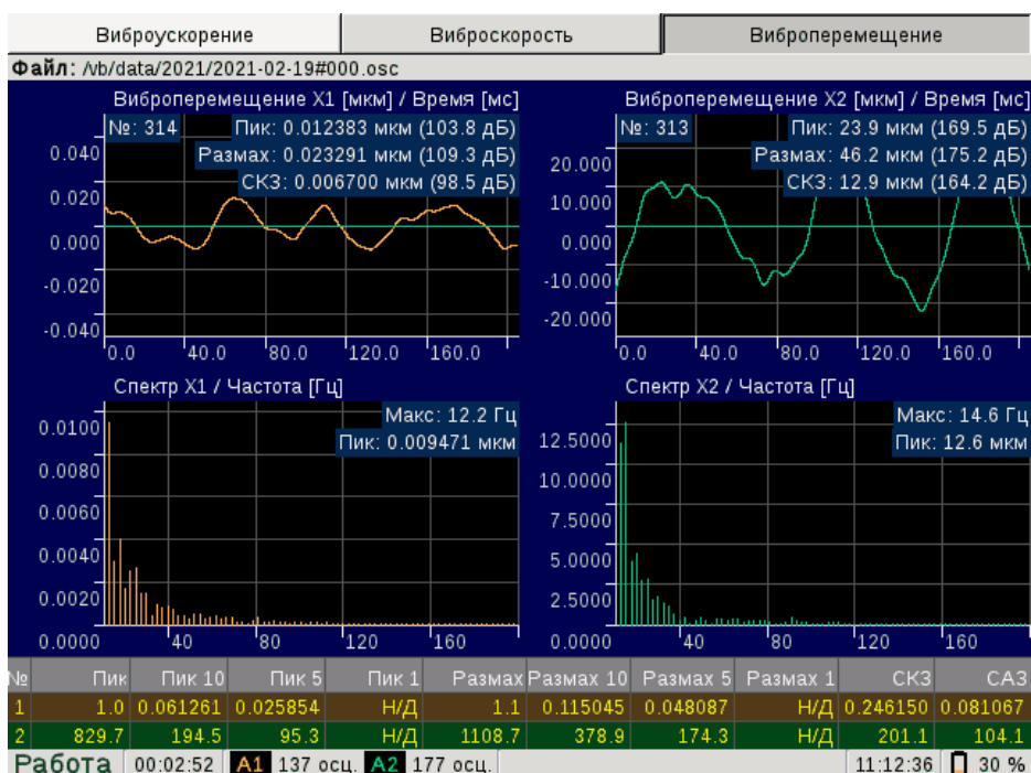
Рис. 5.4. Страница Виброперемещение
